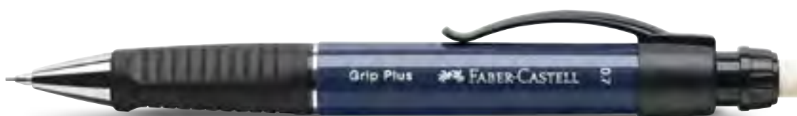
Druckbleistift: Federnd gelagerte 0,7 mm Mine, langer Radierer zum Herausdrehen. Mechanical pencil: mechanical pencil with spring-loaded 0.7 mm lead, twist-out eraser.
